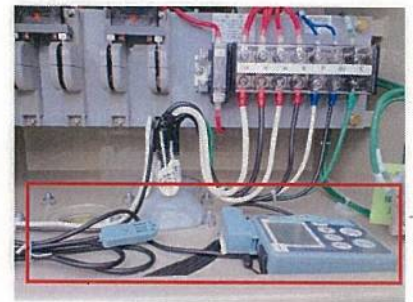
白相内の部温・湿度測定状況 (□が温・湿度計)
